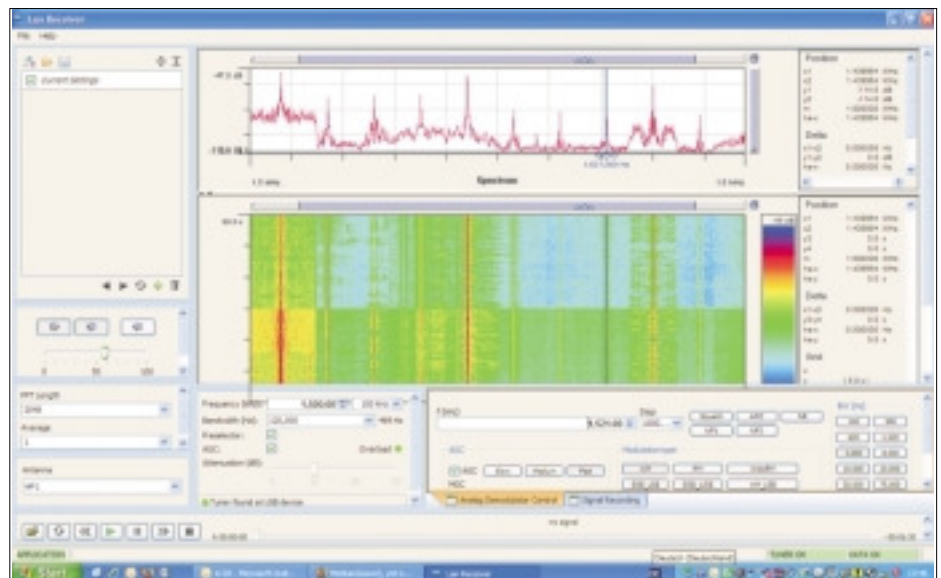
Die virtuelle Frontplatte mit ihren beliebig skalierbaren Teil-Fenstern zeigt hier im Mittelpunkt oben das Spektrum und unten das entsprechende Wasserfalldiagramm eines Mittelwellen-Ausschnittes.
